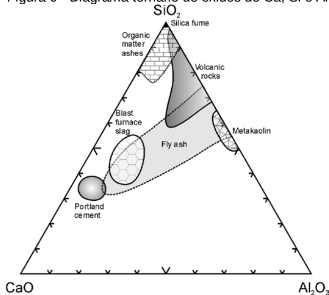
Figura 9 - Diagrama ternário de óxidos de Ca, Si e Al
