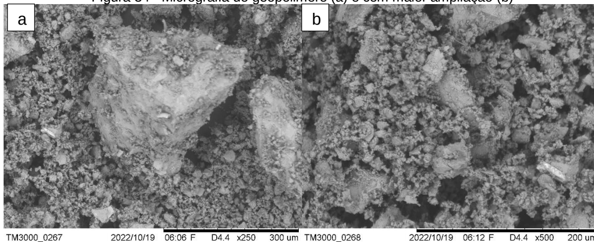
Figura 34 - Micrografia do geopolímero (a) e com maior ampliação (b)
