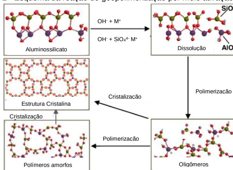
Figura 2 - Esquema da reação de geopolimerização por meio ativação alcalina
