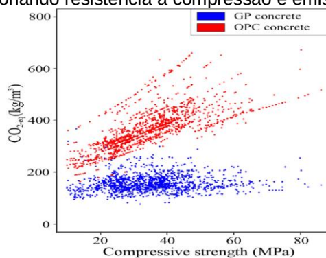
Figura 10 - Gráfico correlacionando resistência à compressão e emissões de gás \text{CO}_2 equivalente
