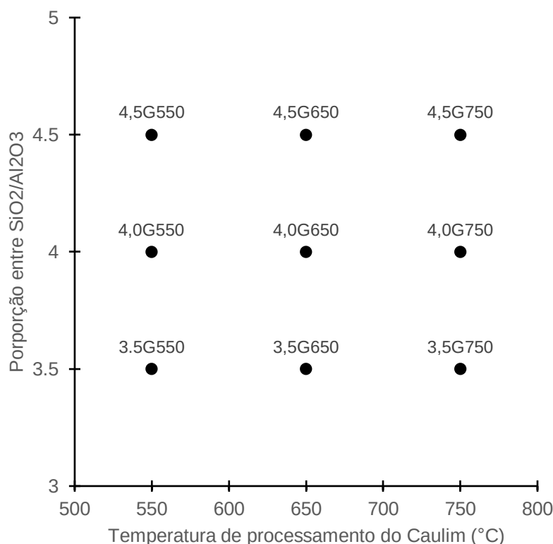
Figura 14 - Pontos de análise para compressão aos 7 dias, dado nas variações de SiO 2 /Al 2 O 3 x Temperatura
