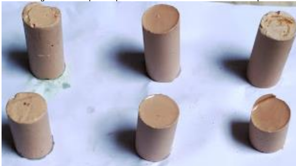
Figura 21 - Corpos de prova desmoldados e antes da retificação
