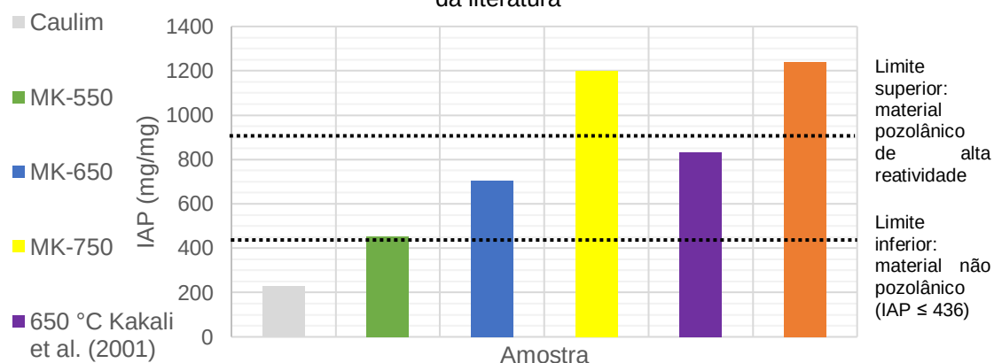
Figura 29 - Comparação entre o índice de atividade pozzolânica deste trabalho com outros dados da literatura
