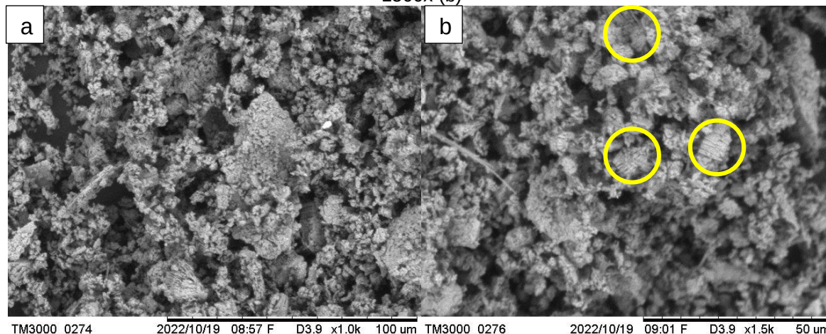
Figura 30 - Morfologia do caulim em 1000x (a) com destaque para aglomerados lamelares em 1500x (b)
