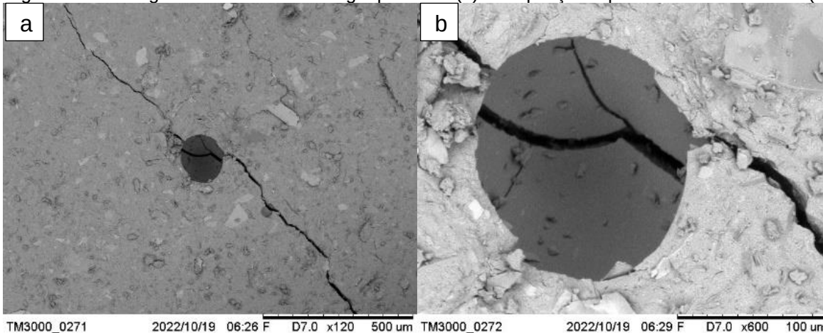
Figura 33 - Micrografia da fratura de um geopolímero (a) e ampliação e porosidade com fratura (b)
