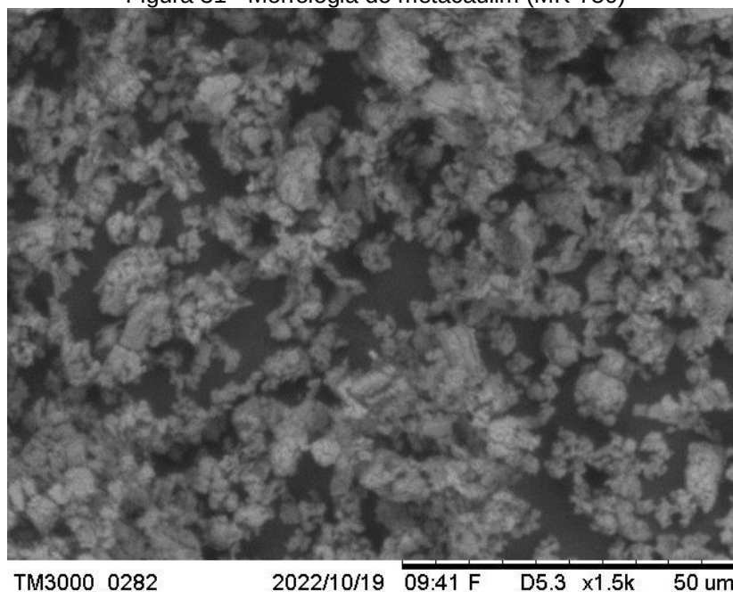
Figura 31 - Morfologia do metacaulim (MK-750)
