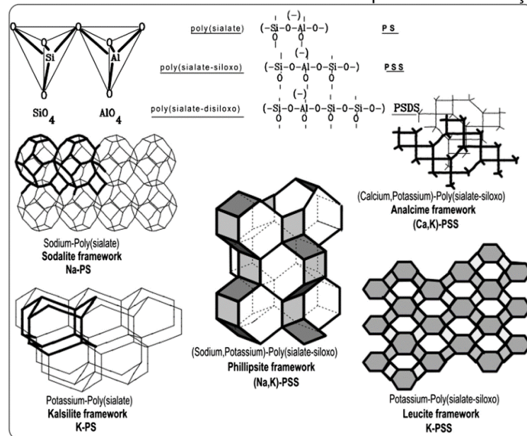
Figura 13 - Possíveis estruturas cristalinas formadas por meio da ativação alcalina
